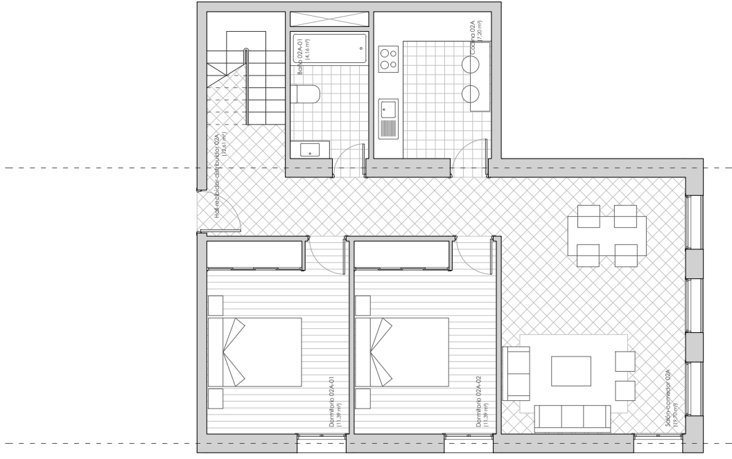
NIVEL INFERIOR DE DÚPLEX
